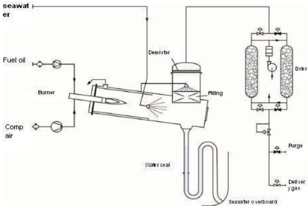
Fig. 1.6. A: Inert gas generator 29
